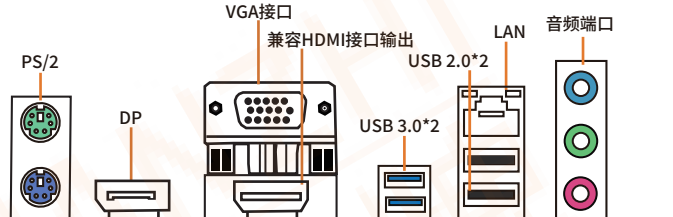
图1-2 整体后置I/O面板展示
