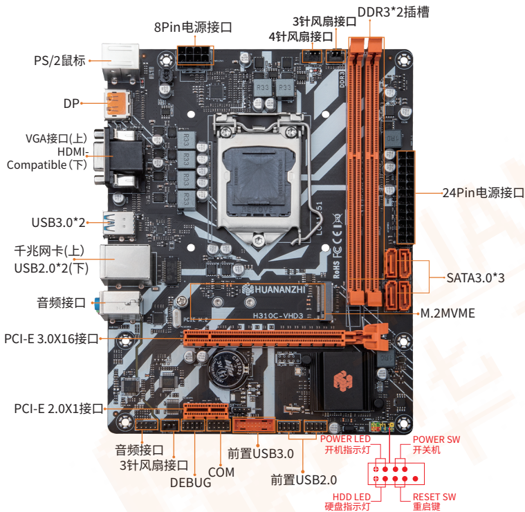
图1-1 H310C-VHD3主板图解
