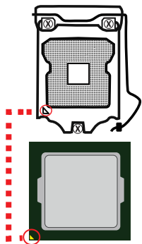
图2-7 CPU安装
